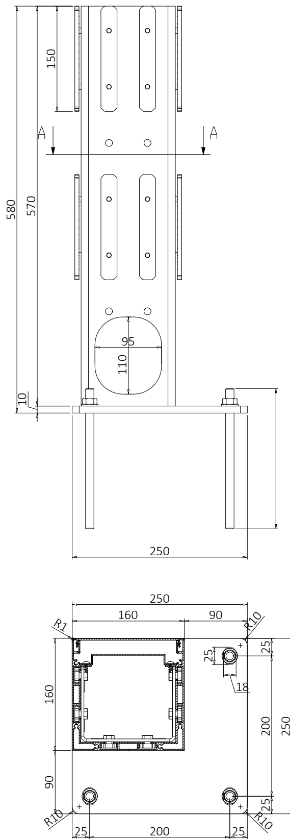
SECTION A-A
